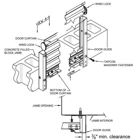
VIEW A-A
